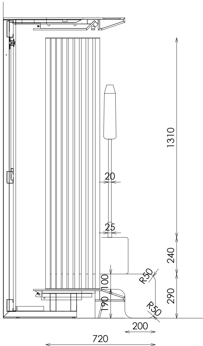
ALZADO LATERAL DERECHO
