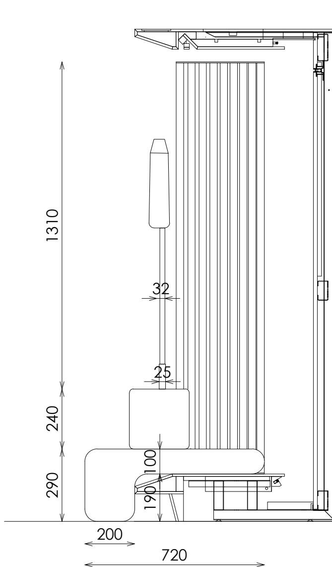
ALZADO LATERAL IZQUIERDO
