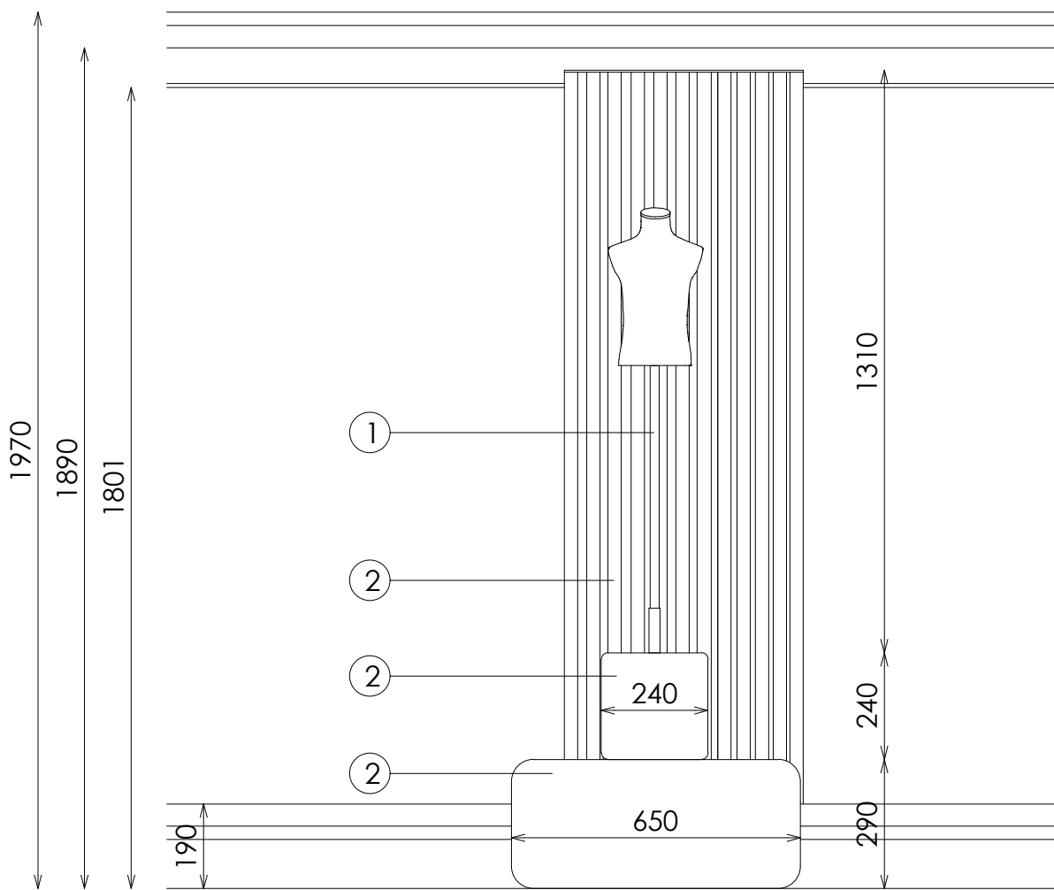
ALZADO FRONTAL
