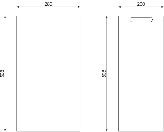
ALZADO FRONTAL
