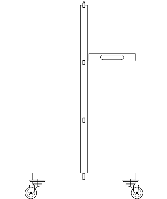
ALZADO LATERAL
