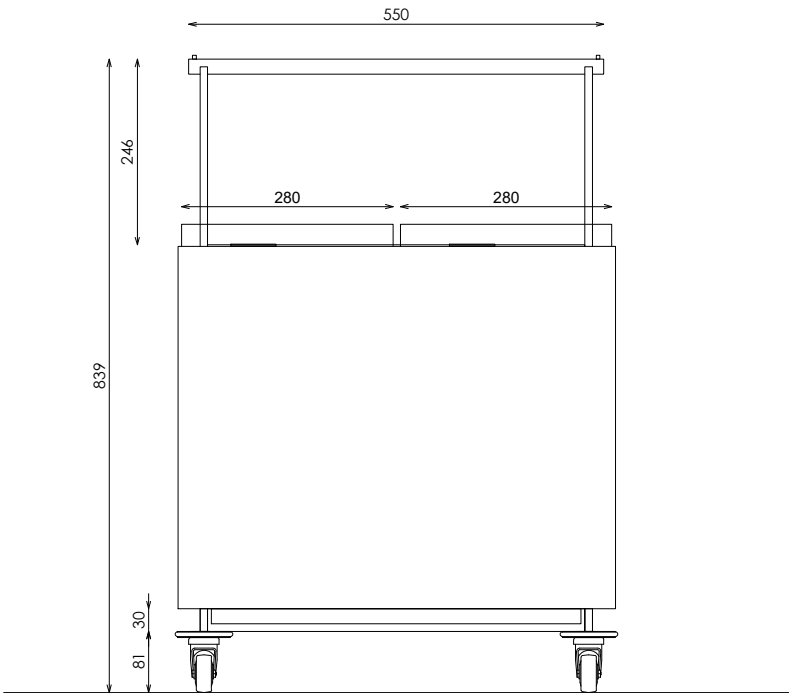
ALZADO FRONTAL
