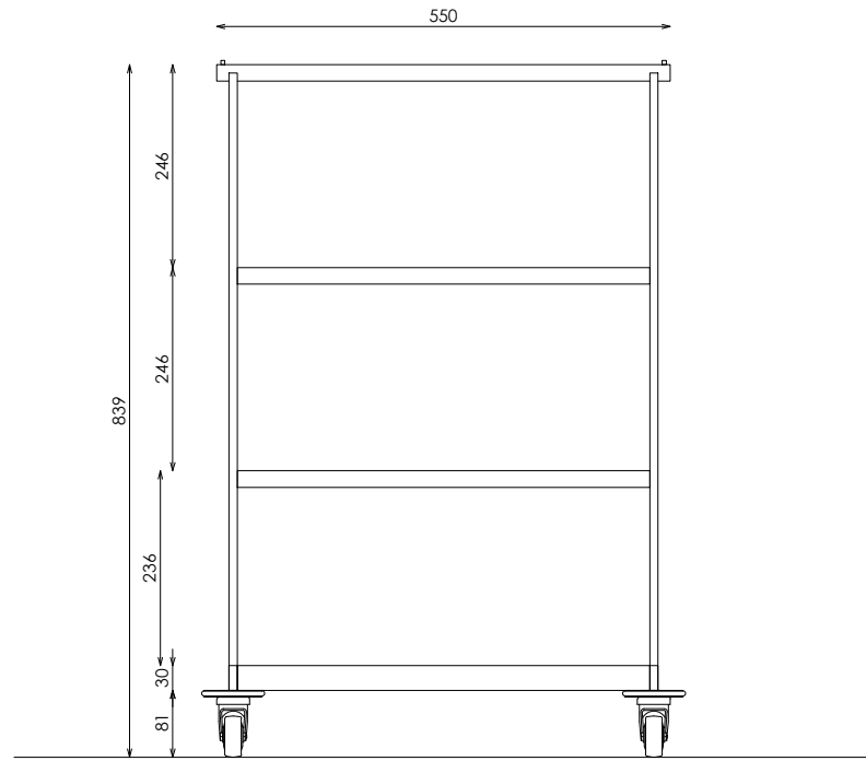
ALZADO FRONTAL
