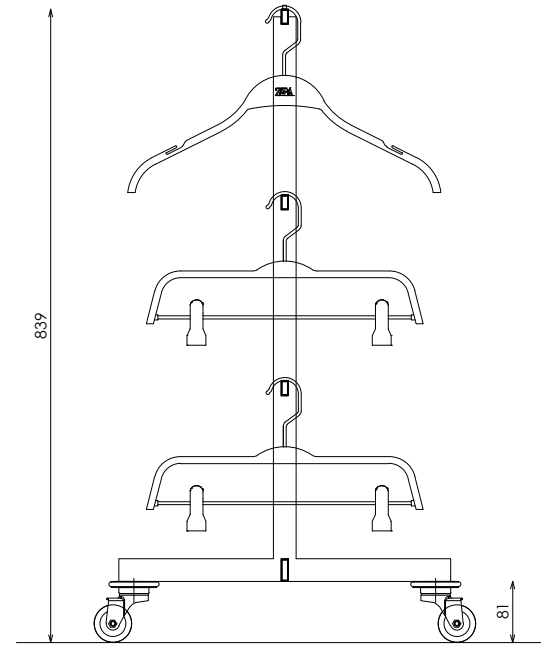
ALZADO LATERAL
