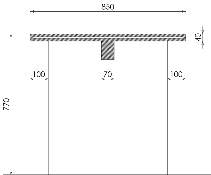
SECCION LATERAL
