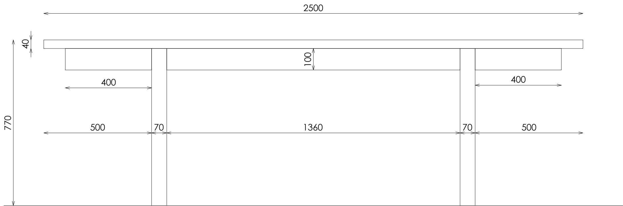
ALZADO FRONTAL
