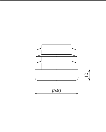
DET. CONTERAS
