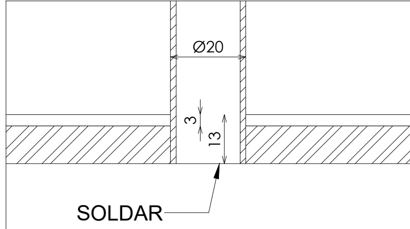
DETALLE C
