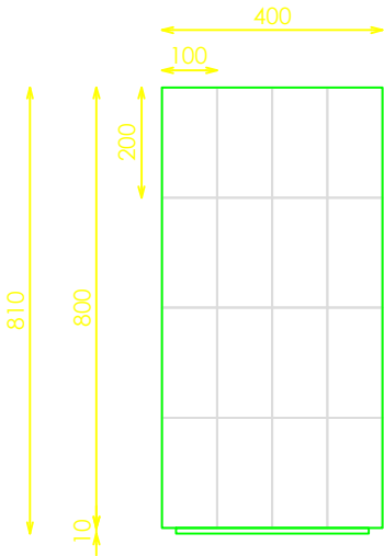
ALZADO
