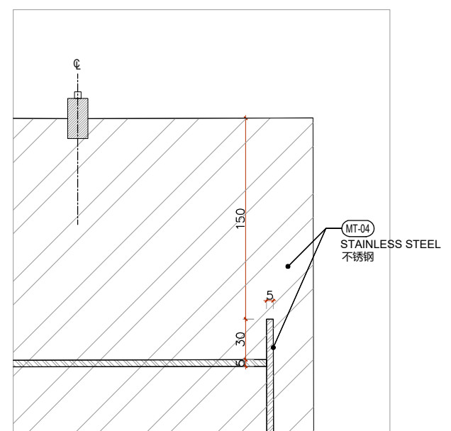
6 节点 1:2 DETAIL
