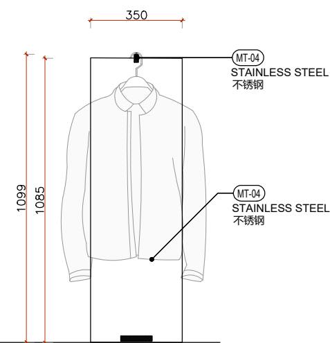
3 侧立面 1:10 SIDE ELEVATION
