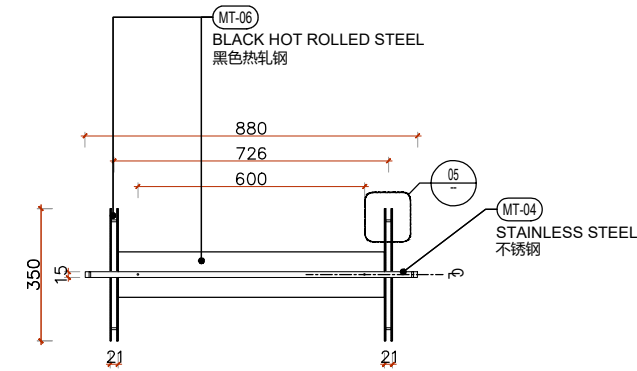
1 平面图 1:10 PLAN
