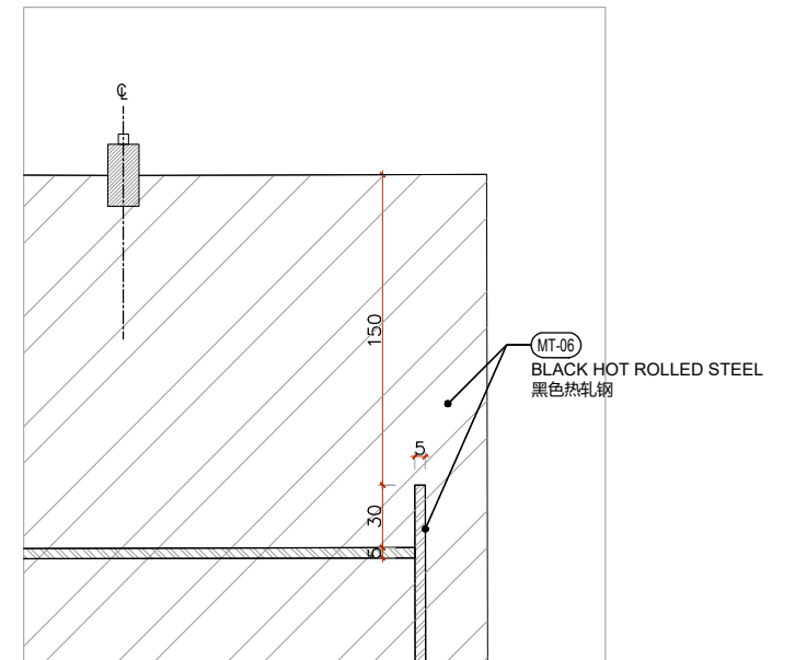
6 节点 1:2 DETAIL
