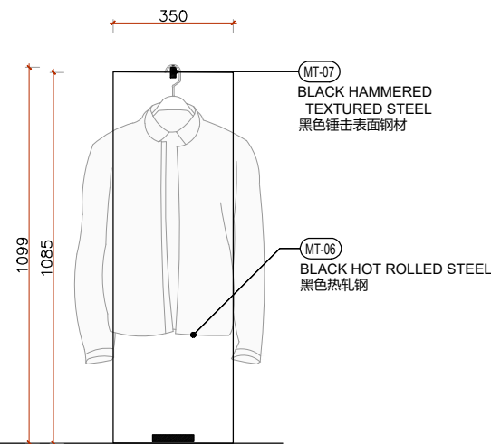
3 侧立面 1:10 SIDE ELEVATION
