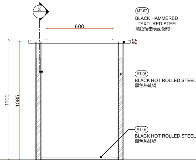
2 正立面 1:10 FRONT ELEVATION
