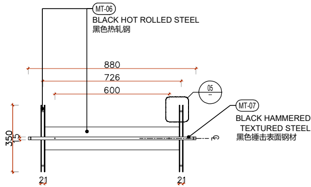
1 平面图 1:10 PLAN
