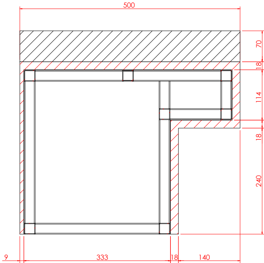
剖面 AJ-AJ 比例 1 : 5
