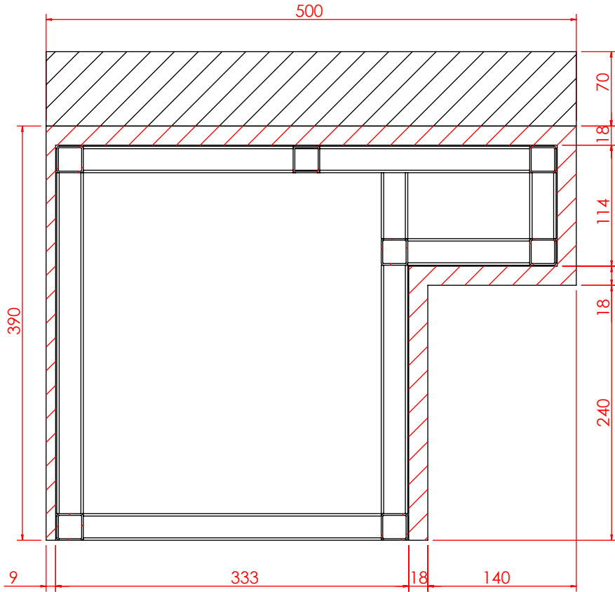
剖面 AJ-AJ 比例 1 : 5
