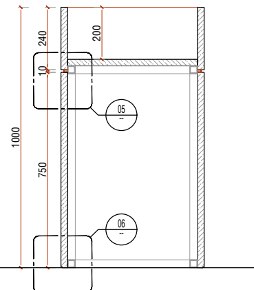
4 剖面 1:10 SECTION
