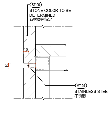
5 节点 01 1:2 DETAIL 01
