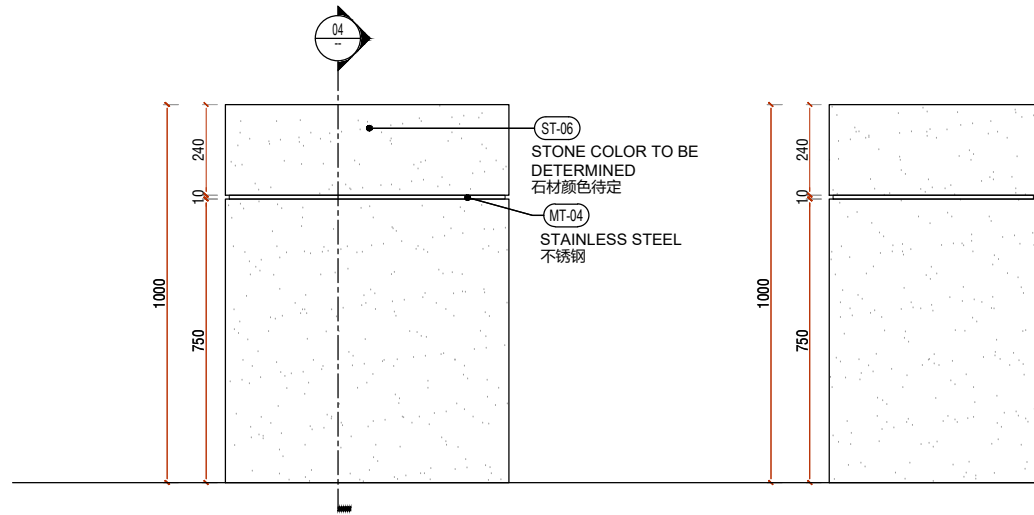
1 平面图 1:10 PLAN
