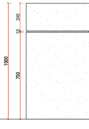
3 侧立面 1:10 SIDE ELEVATION
