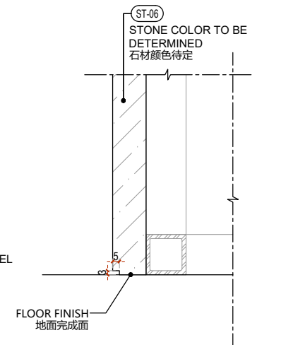
6 节点 01 1:2 DETAIL 01
