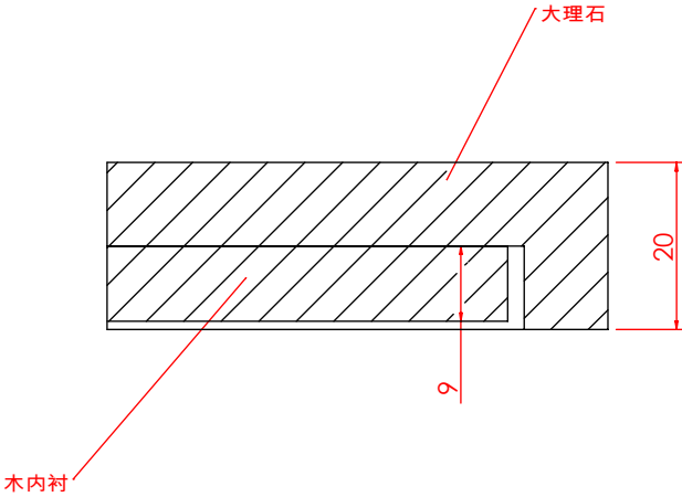
局部视图 B 比例 1 : 1
