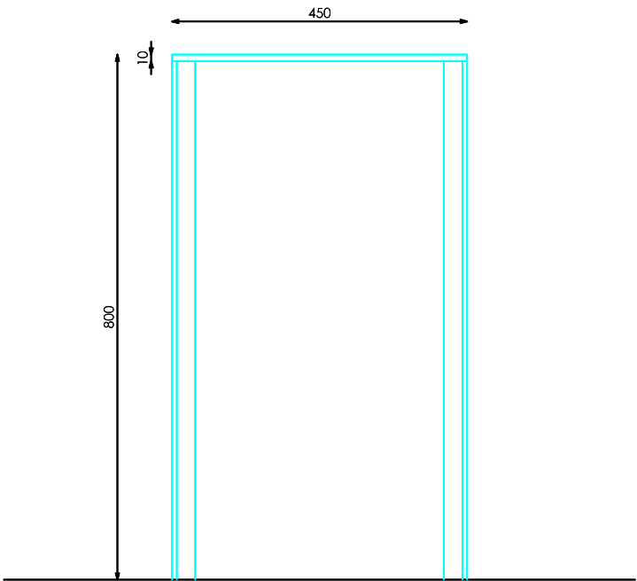
ALZADO LATERAL
