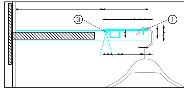
BARRA CUELGA. DETALLE
