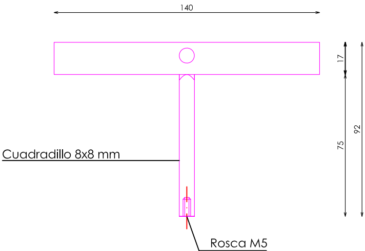
ALZADO
