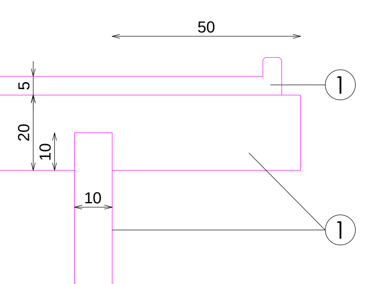
DETALLE C
