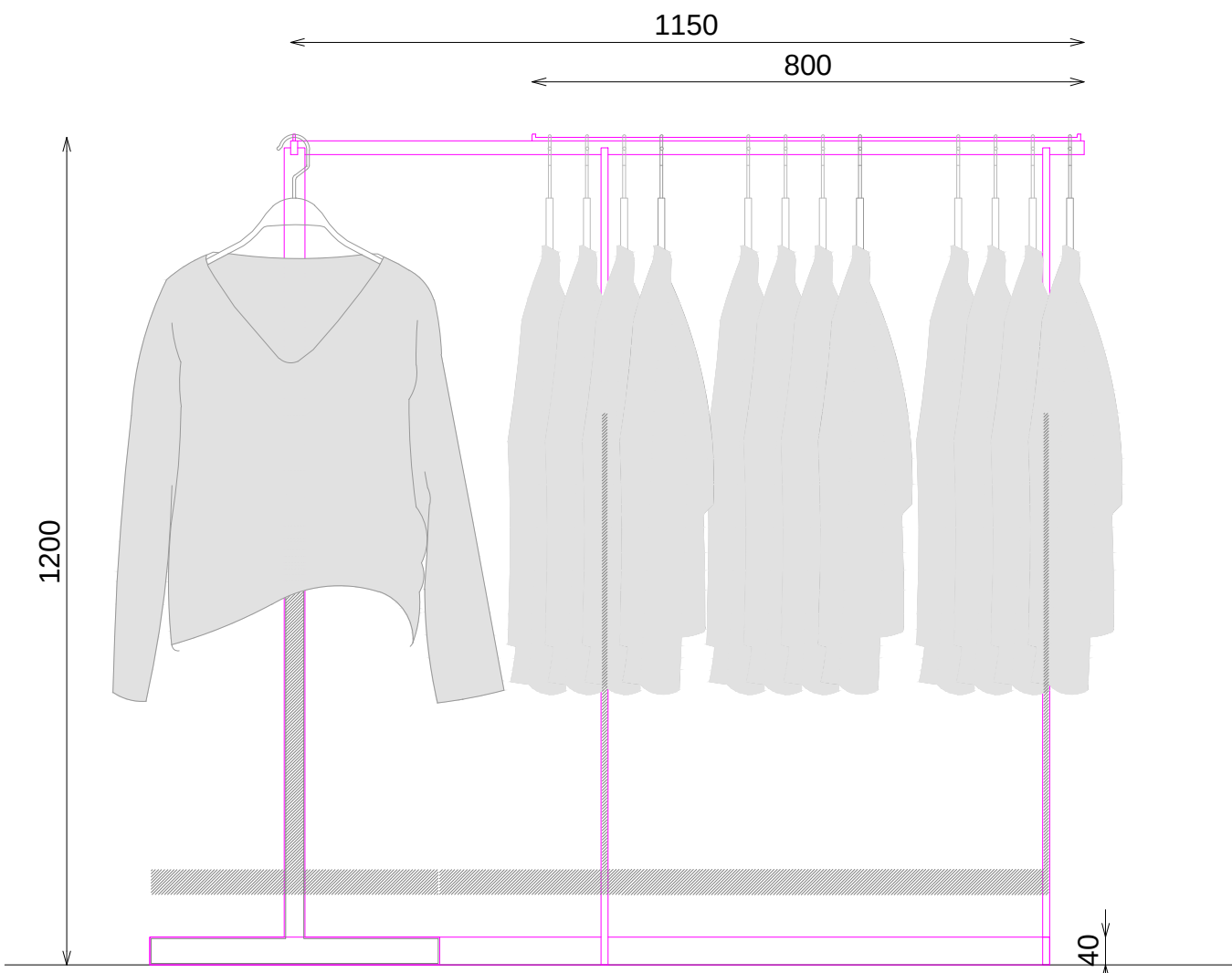
ALZADO FRONTAL
