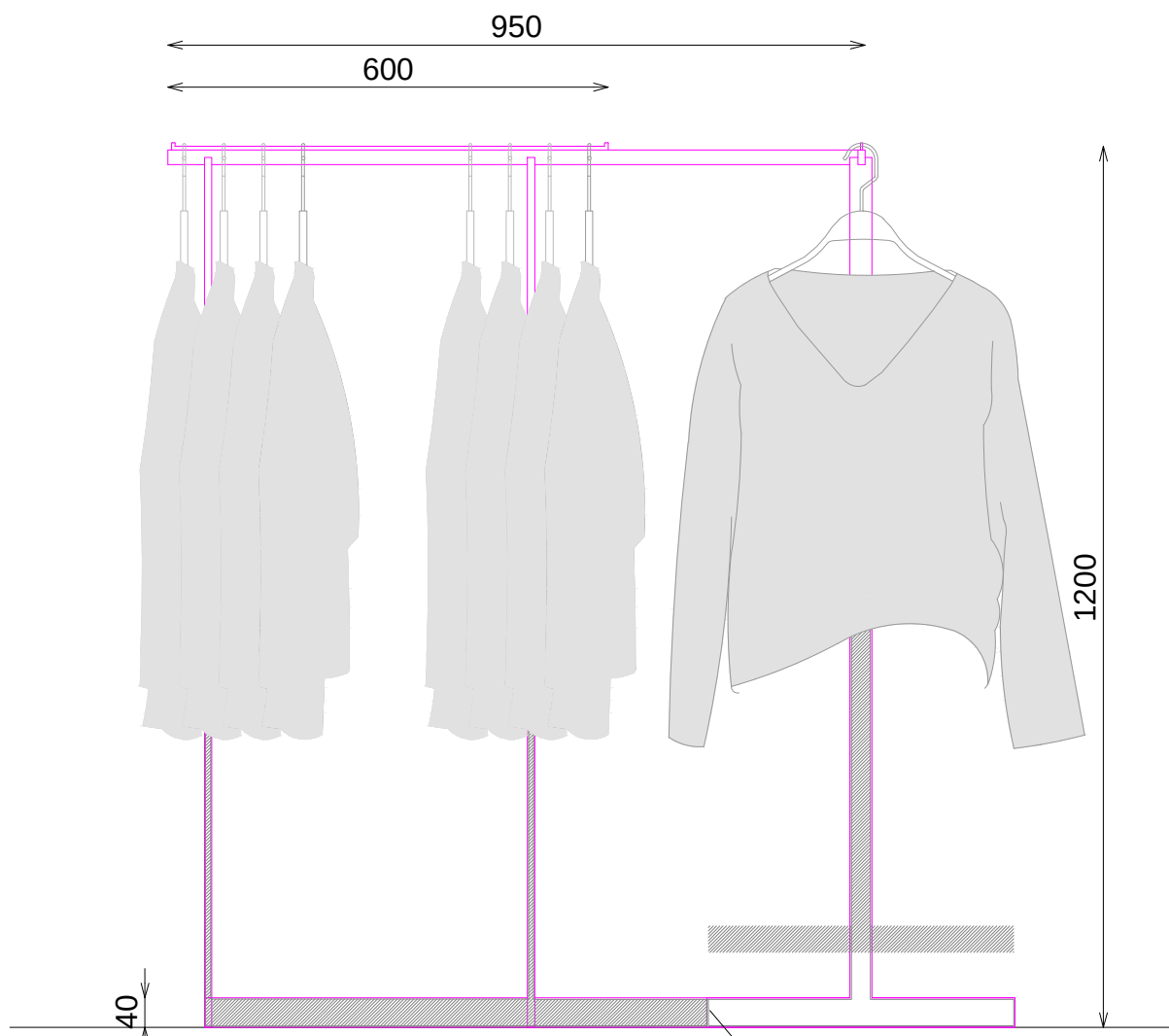
ALZADO LATERAL
