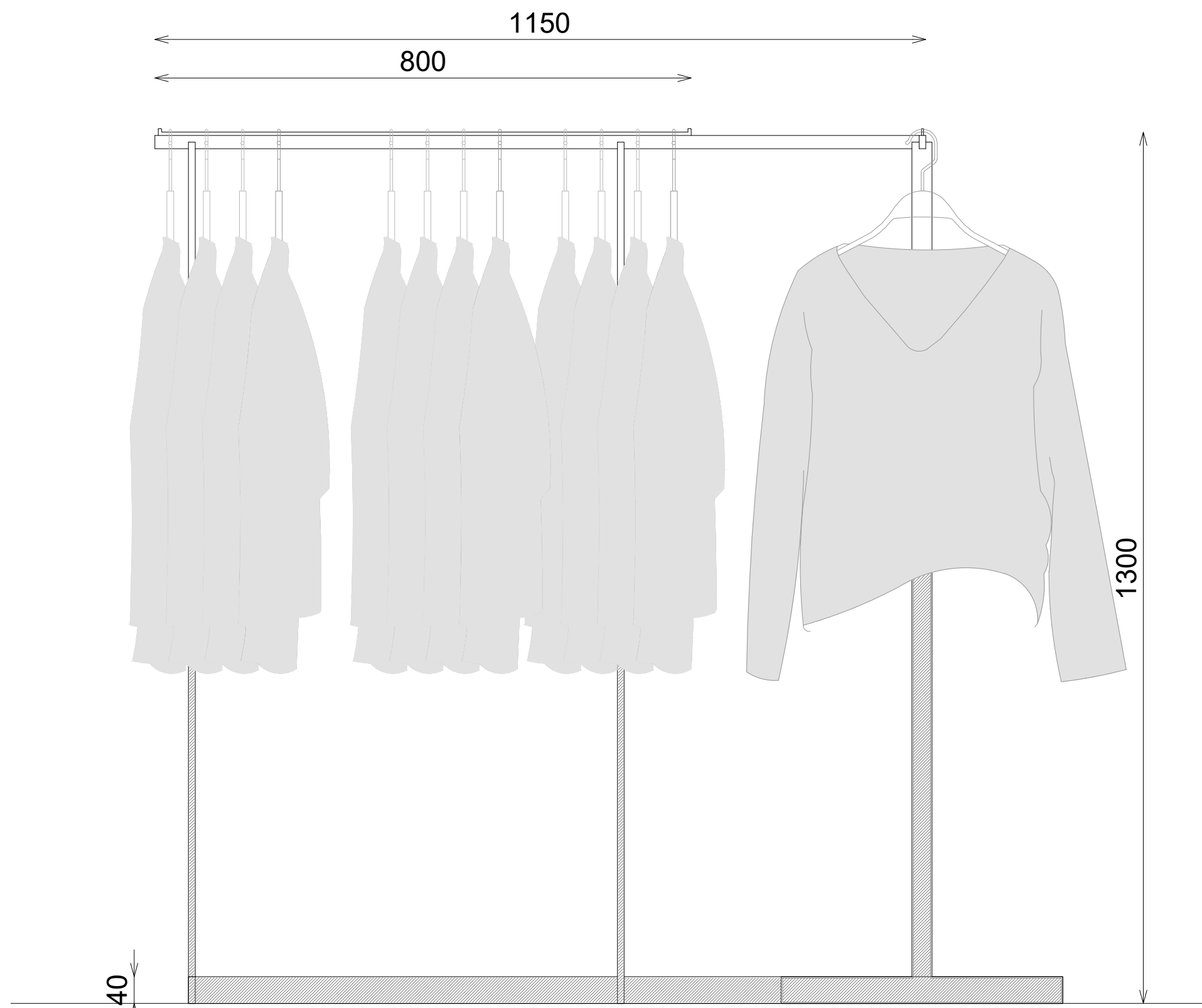
ALZADO FRONTAL
