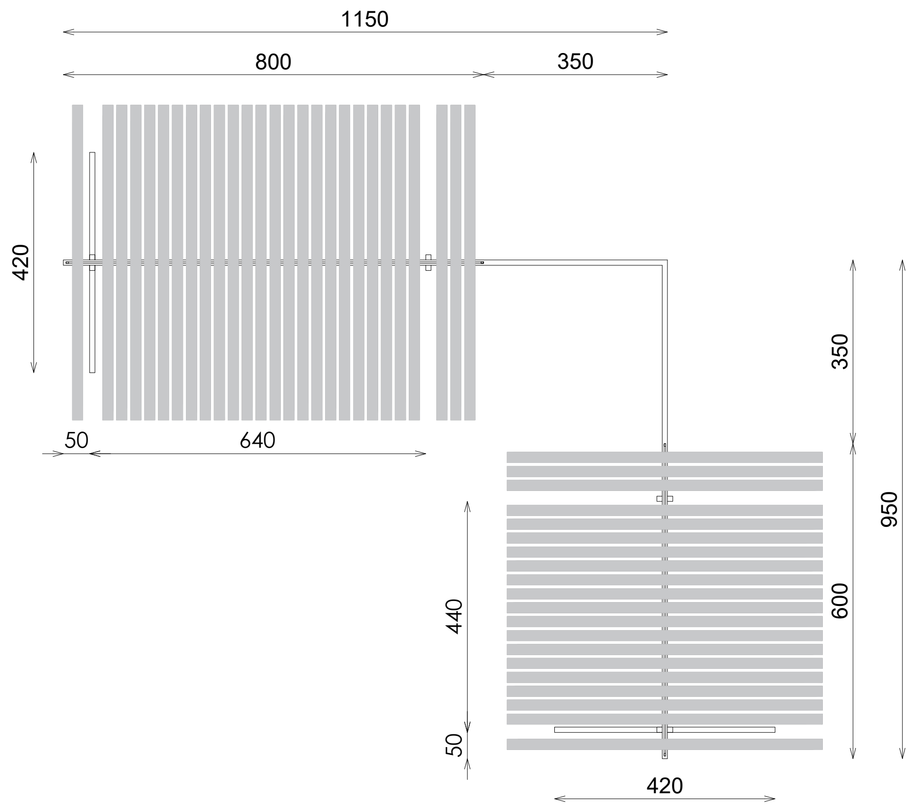
PLANTA
