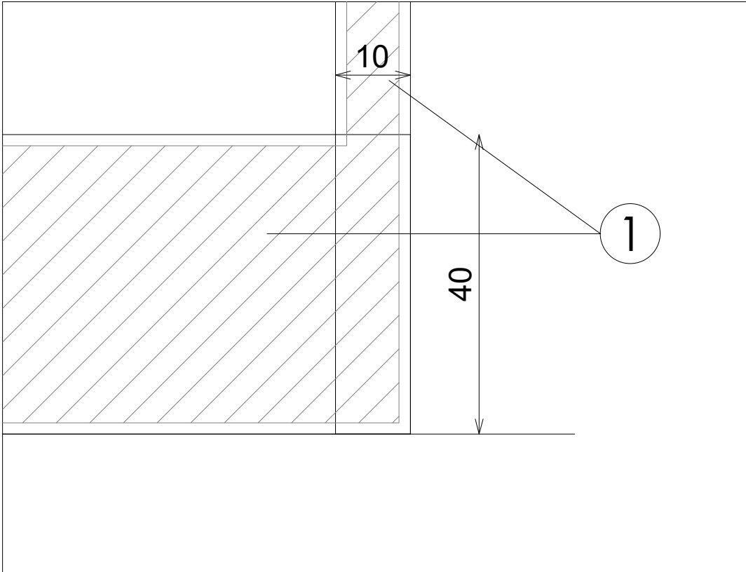
DETALLE C
