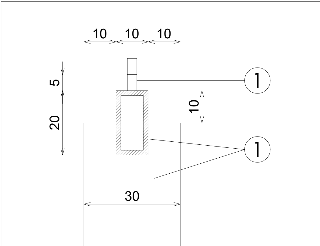
DETALLE A
