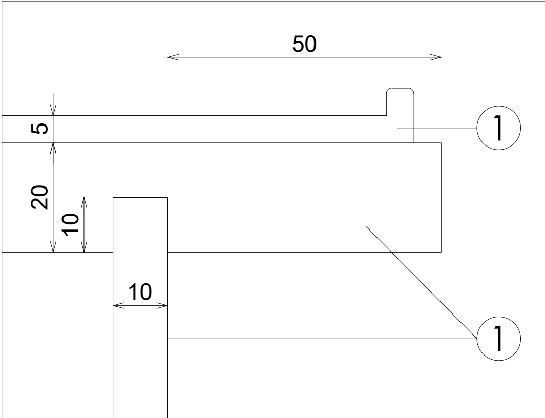
DETALLE B
