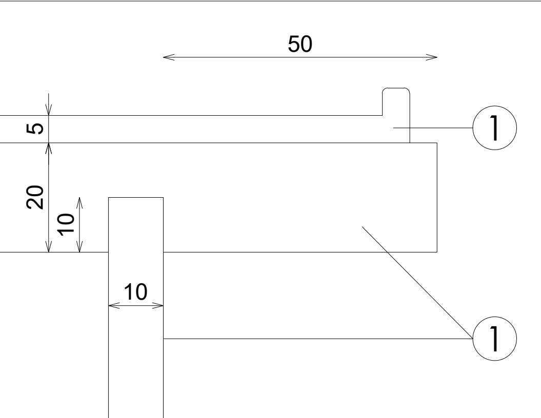
DETALLE C
