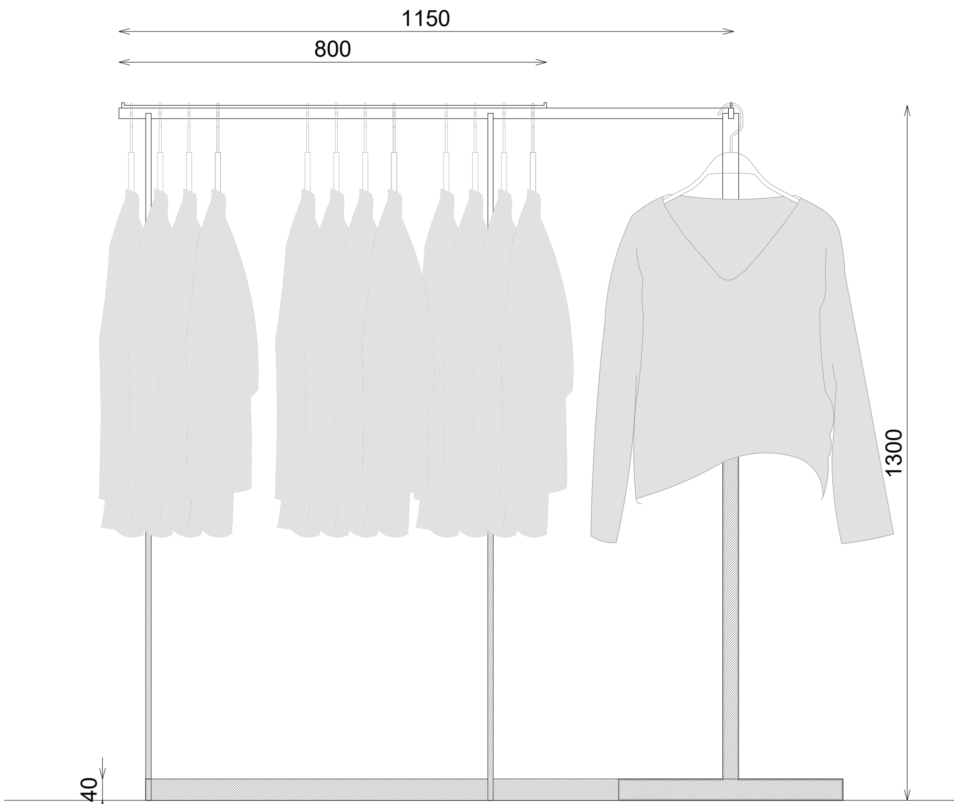
ALZADO FRONTAL
