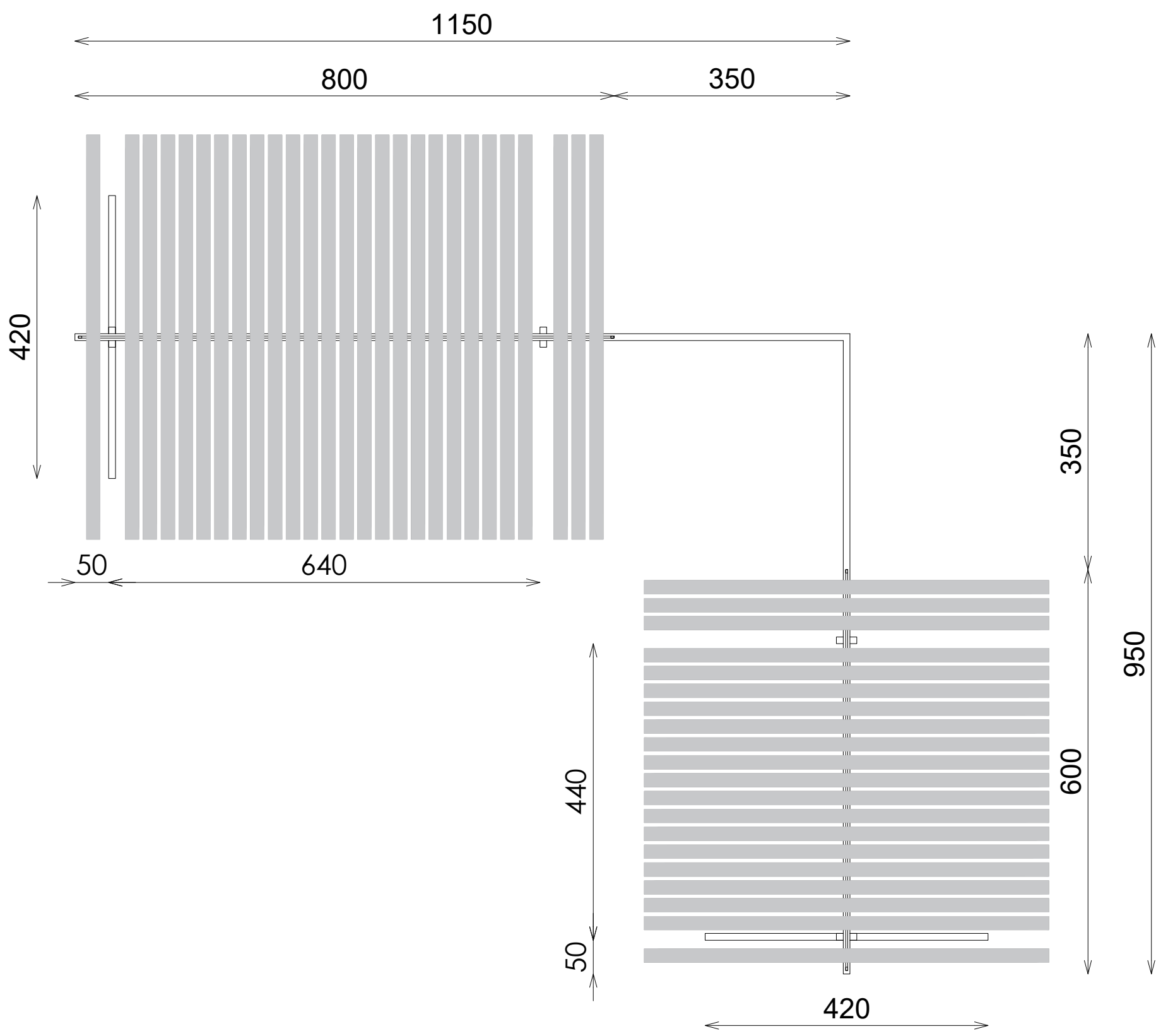
PLANTA
