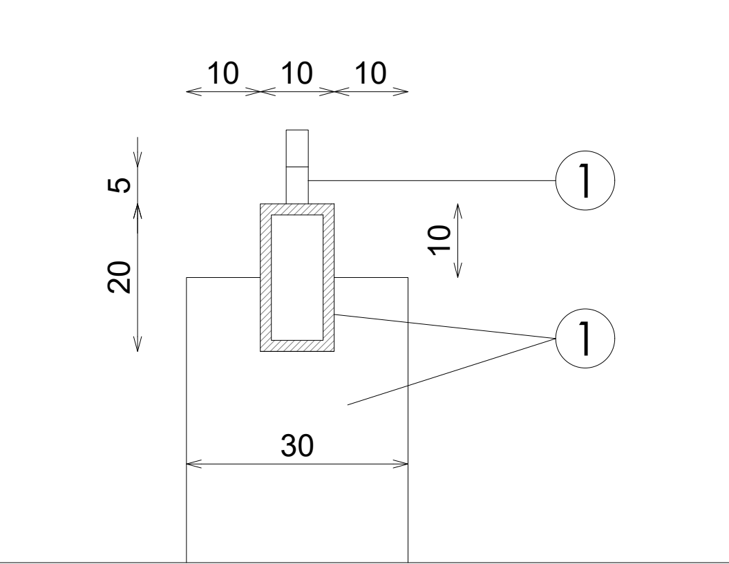
DETALLE B
