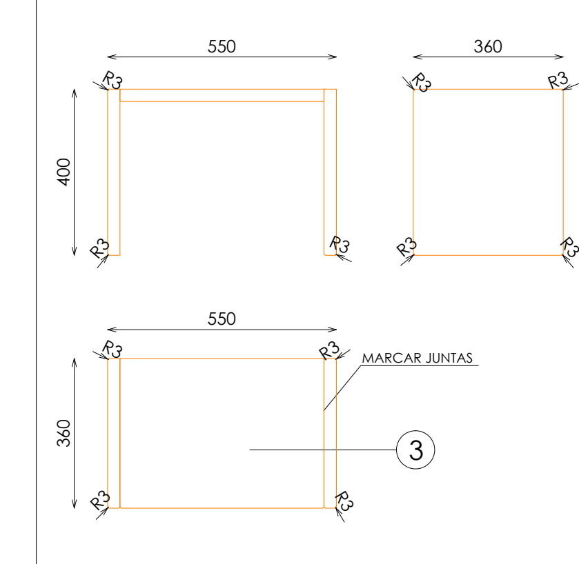
BANCO CURVO 55
