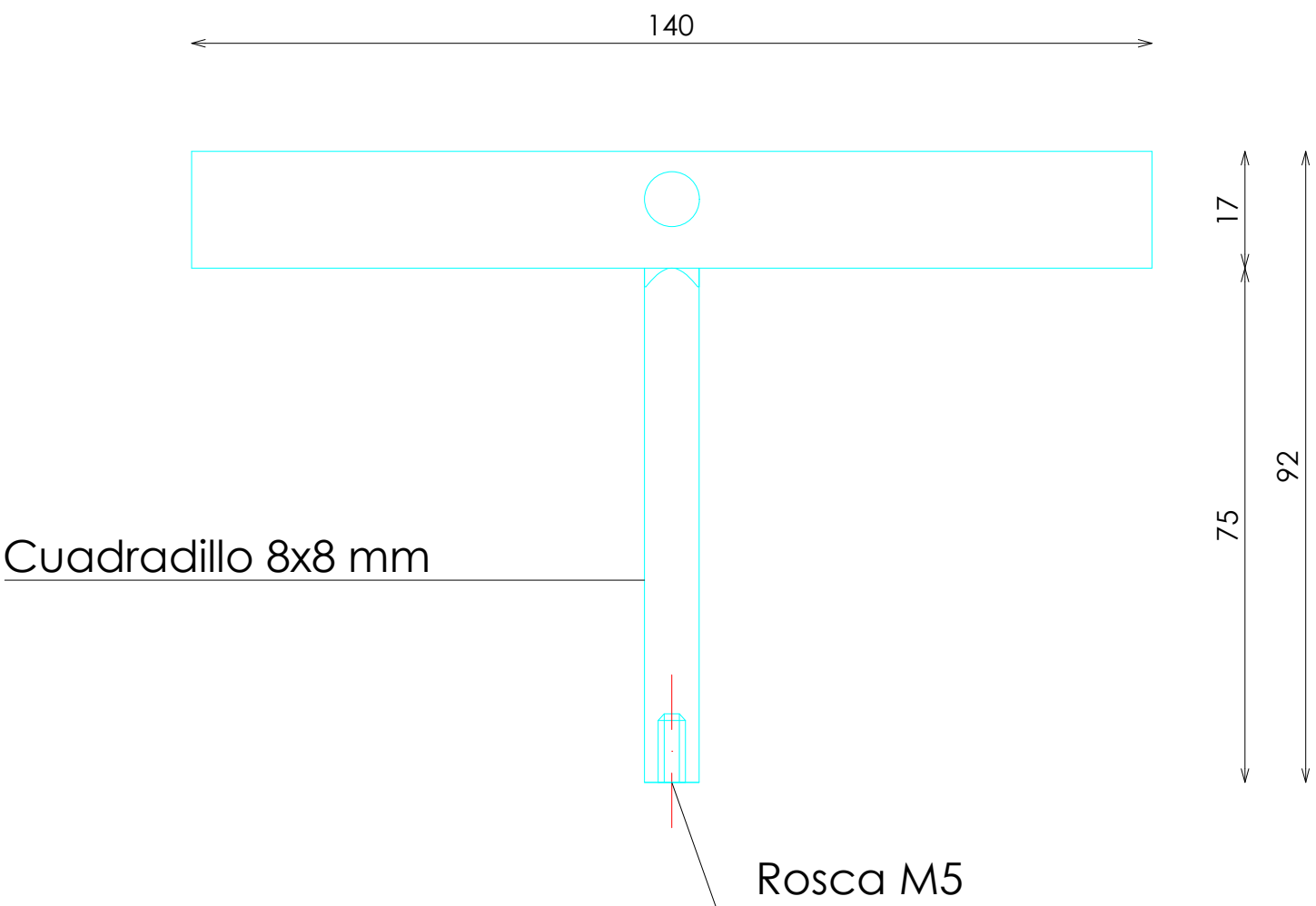
ALZADO
