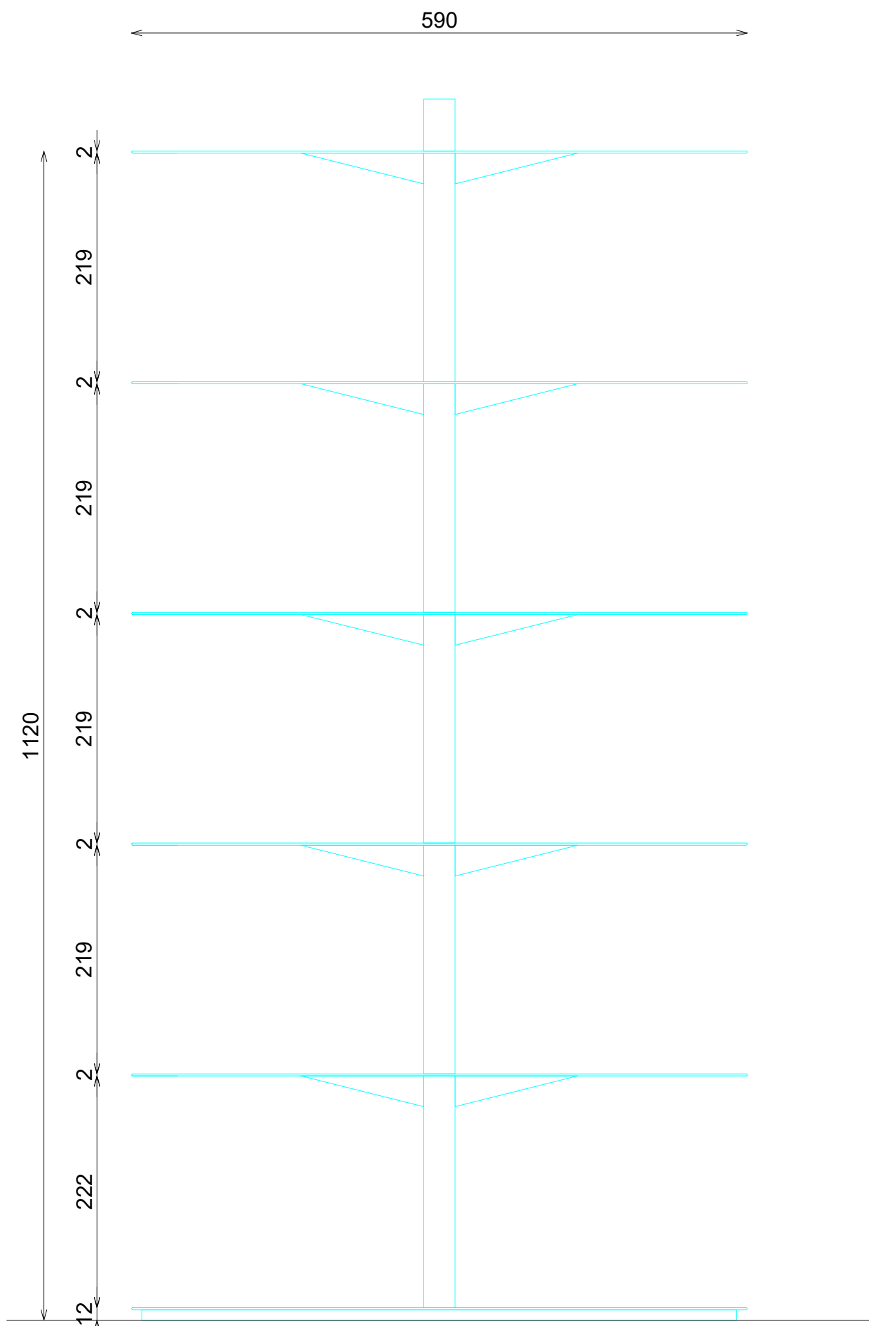
ALZADO
