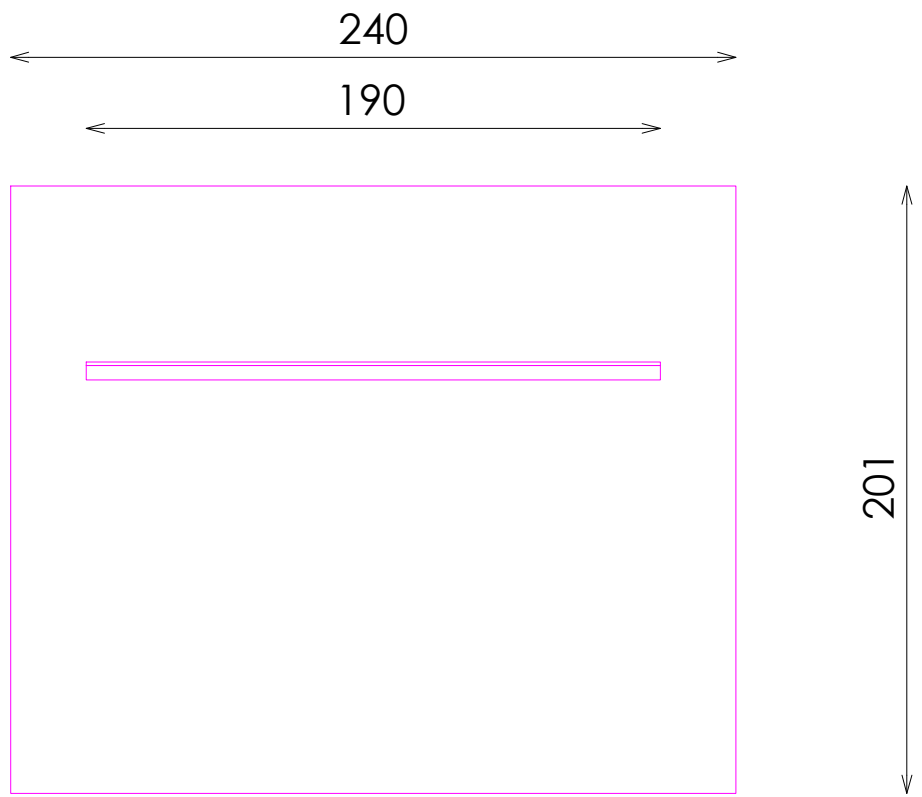
ALZADO
