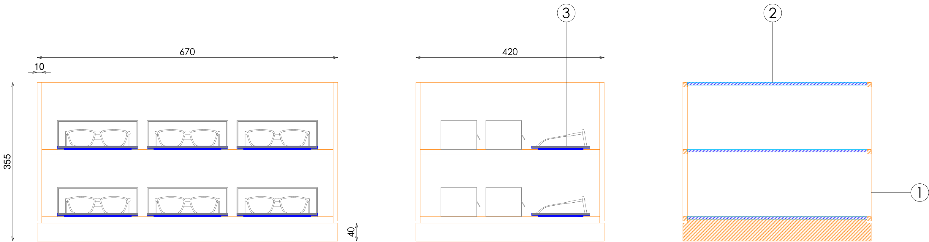
ALZADO
