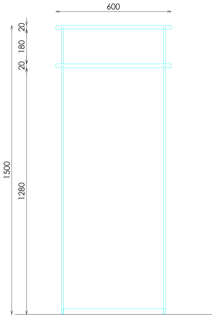
ALZADO
