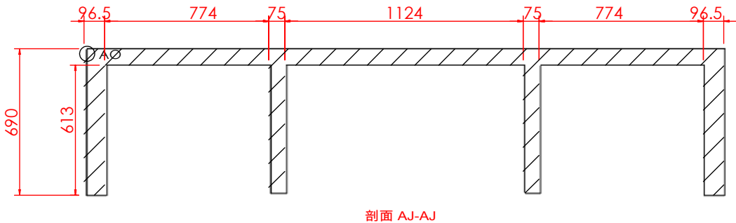
剖面 AJ-AJ
