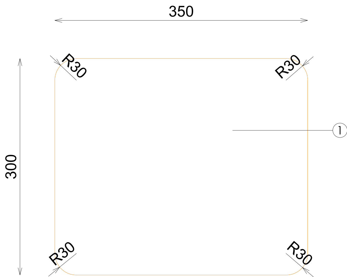
PLANTA
