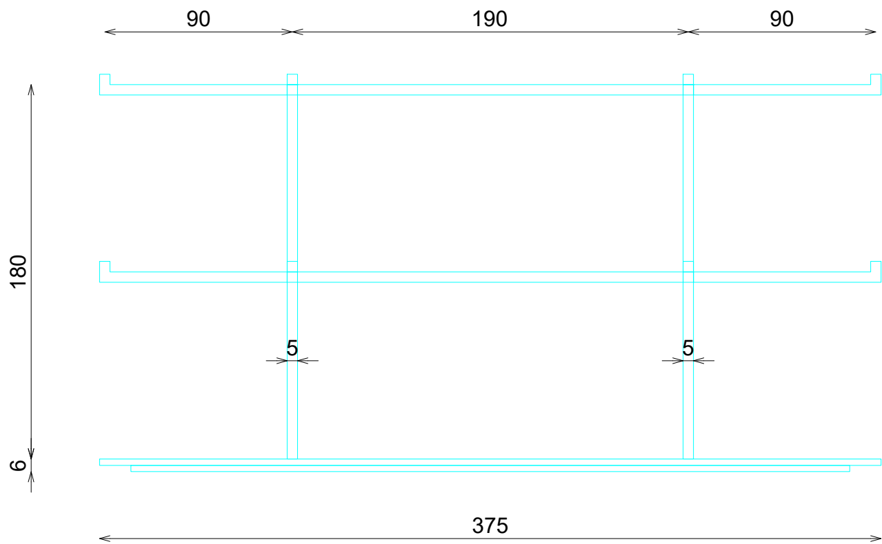
ALZADO
