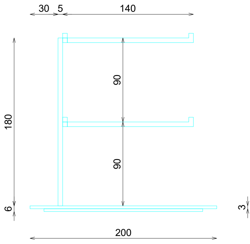
PERFIL
