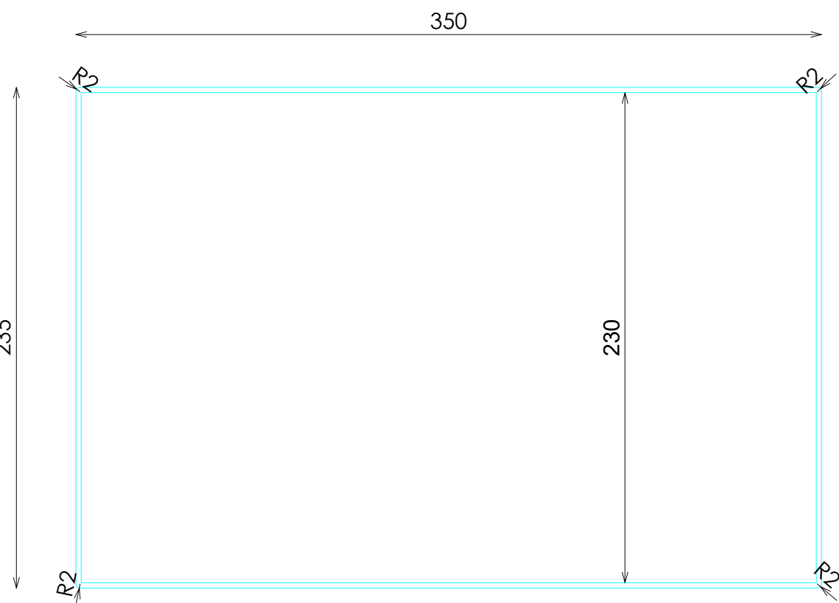
PLANTA
