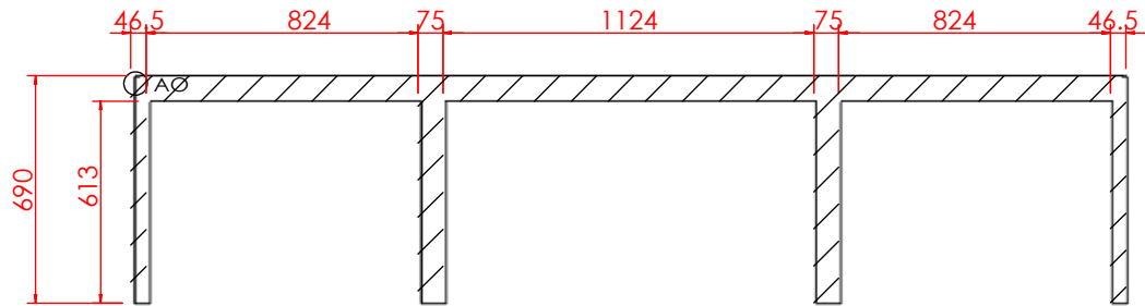
剖面 AJ-AJ
