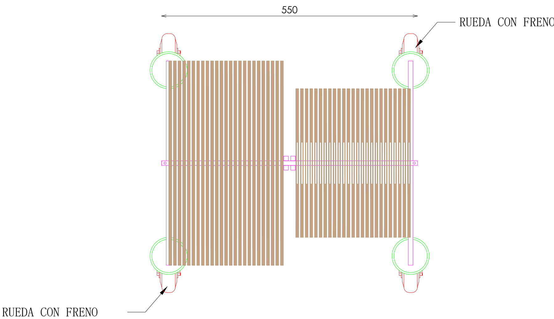
PLANTA
