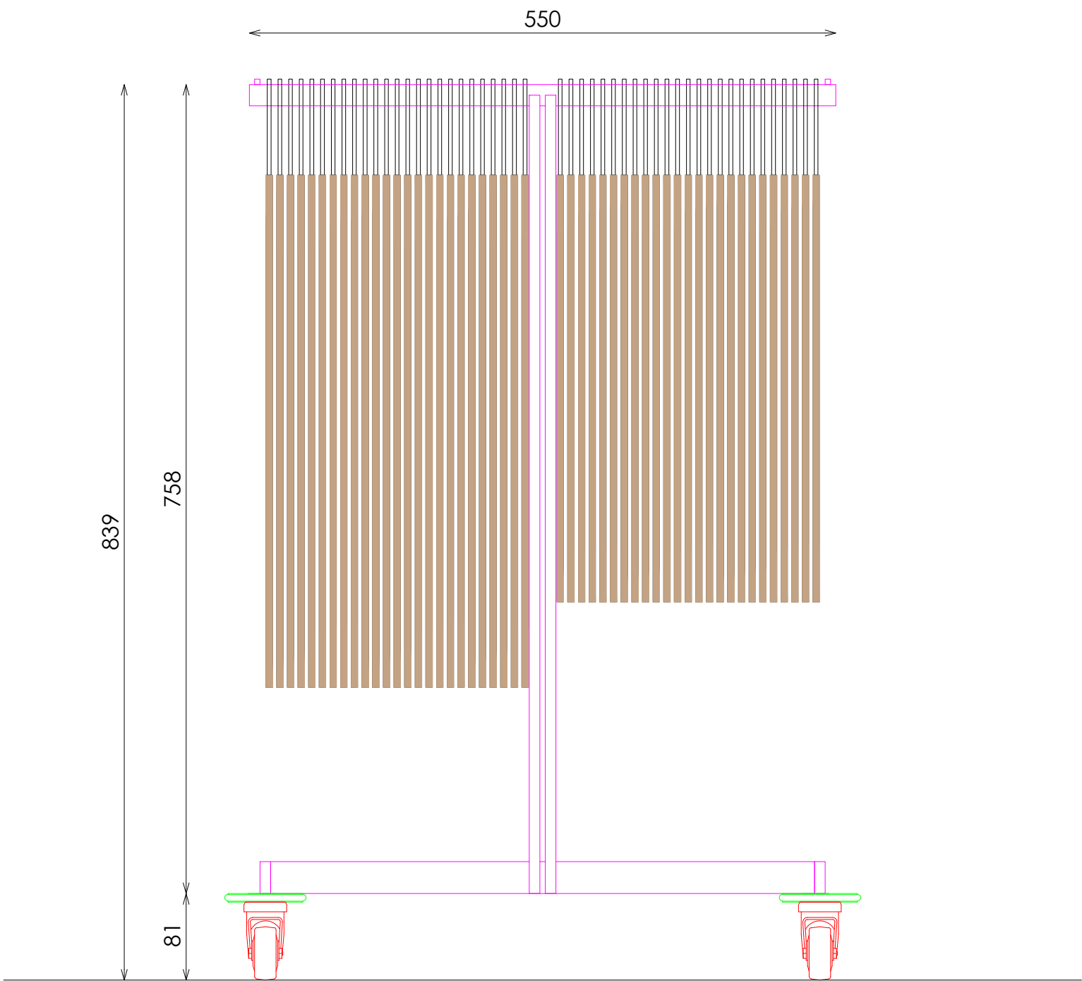
ALZADO FRONTAL
