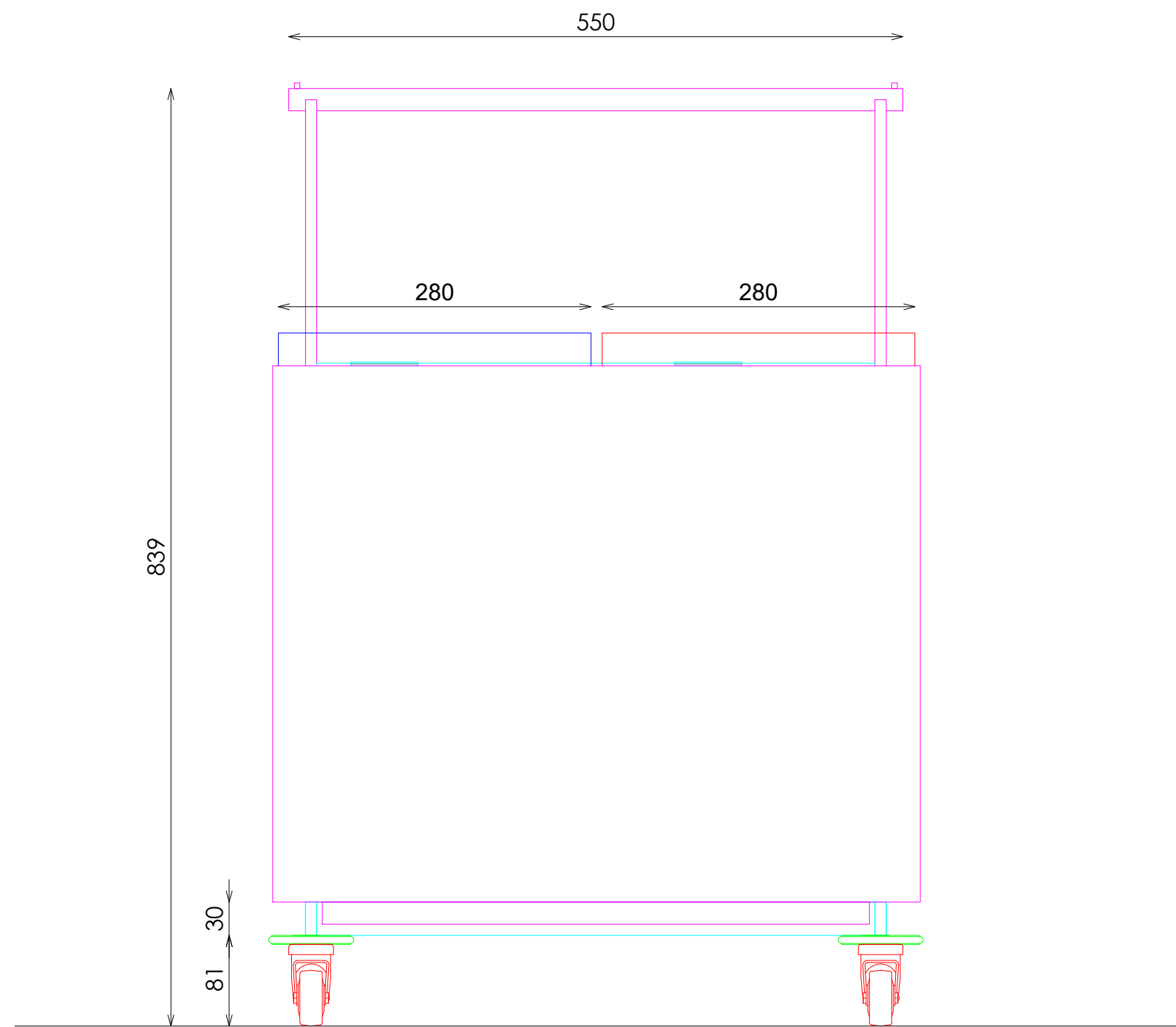
ALZADO FRONTAL
