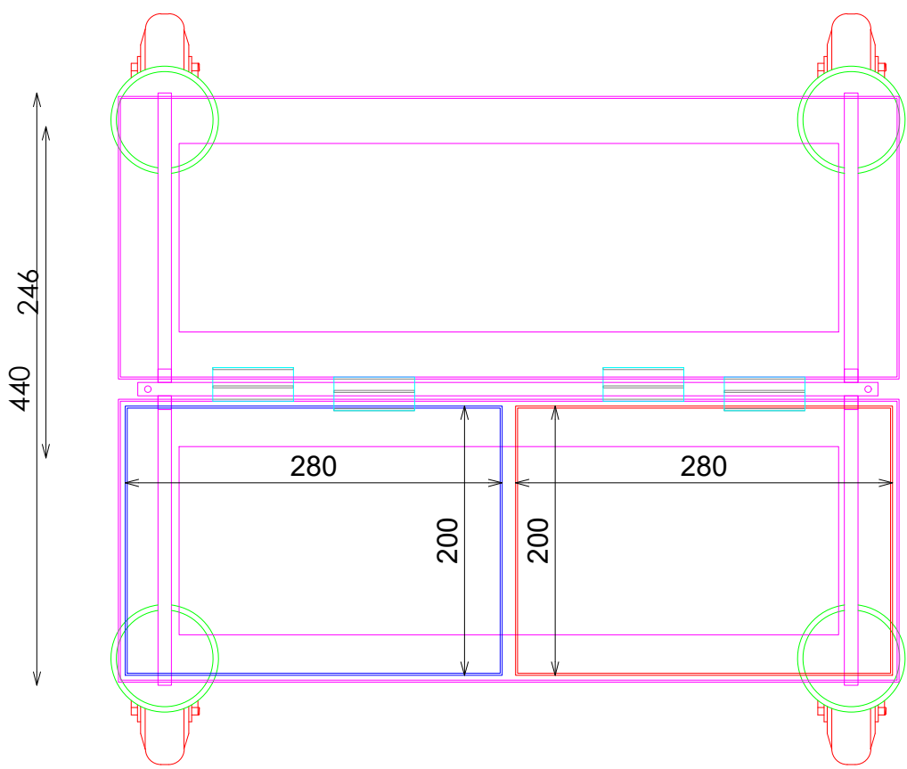
PLANTA
