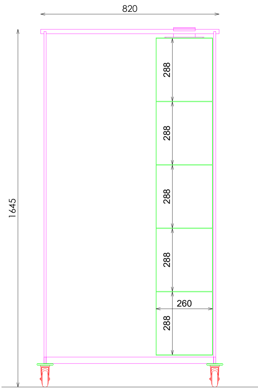
ALZADO
