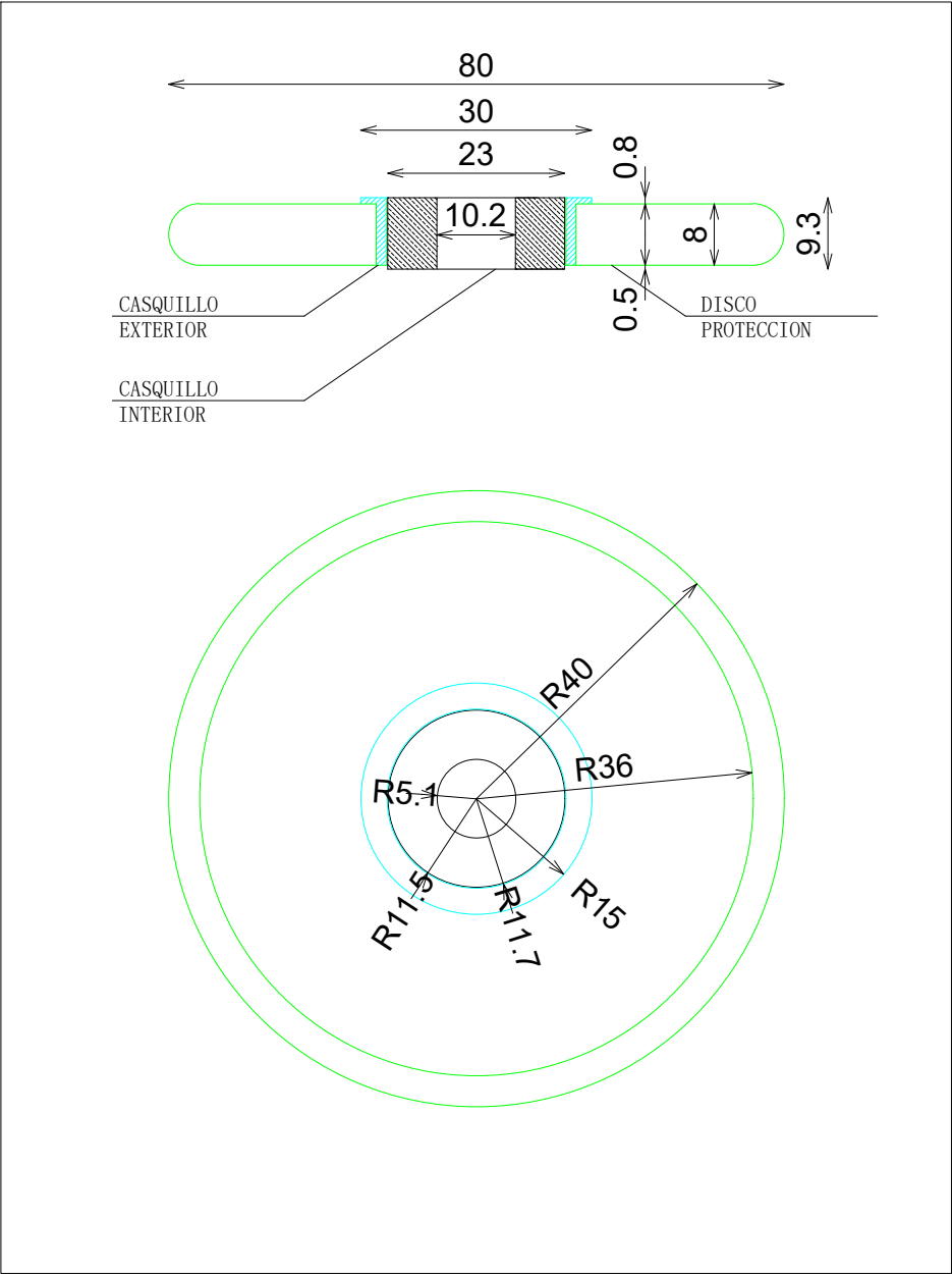
DETALLE DISCO PROTECCION
