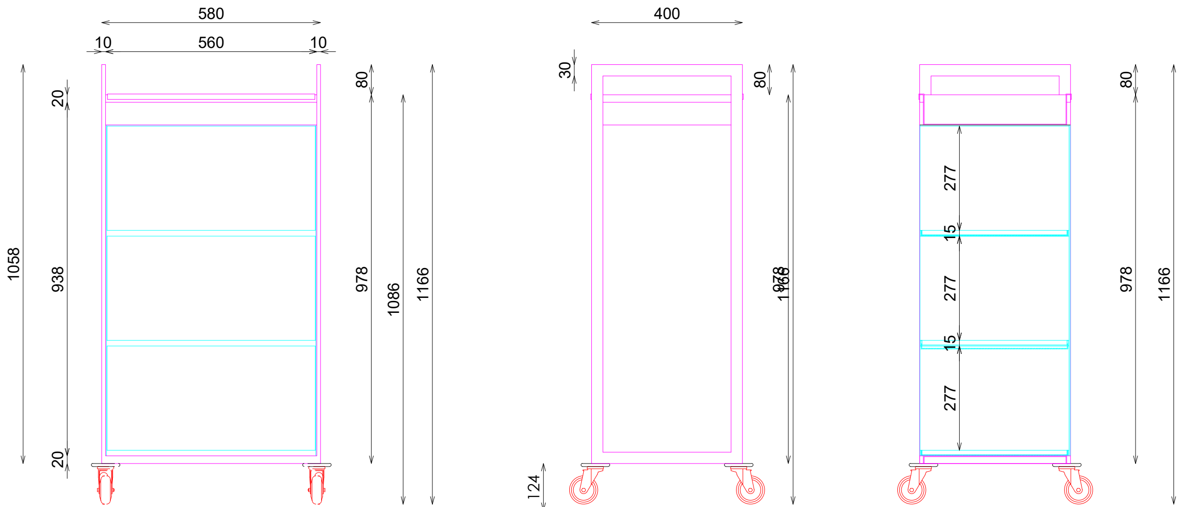
ALZADO FRONTAL
