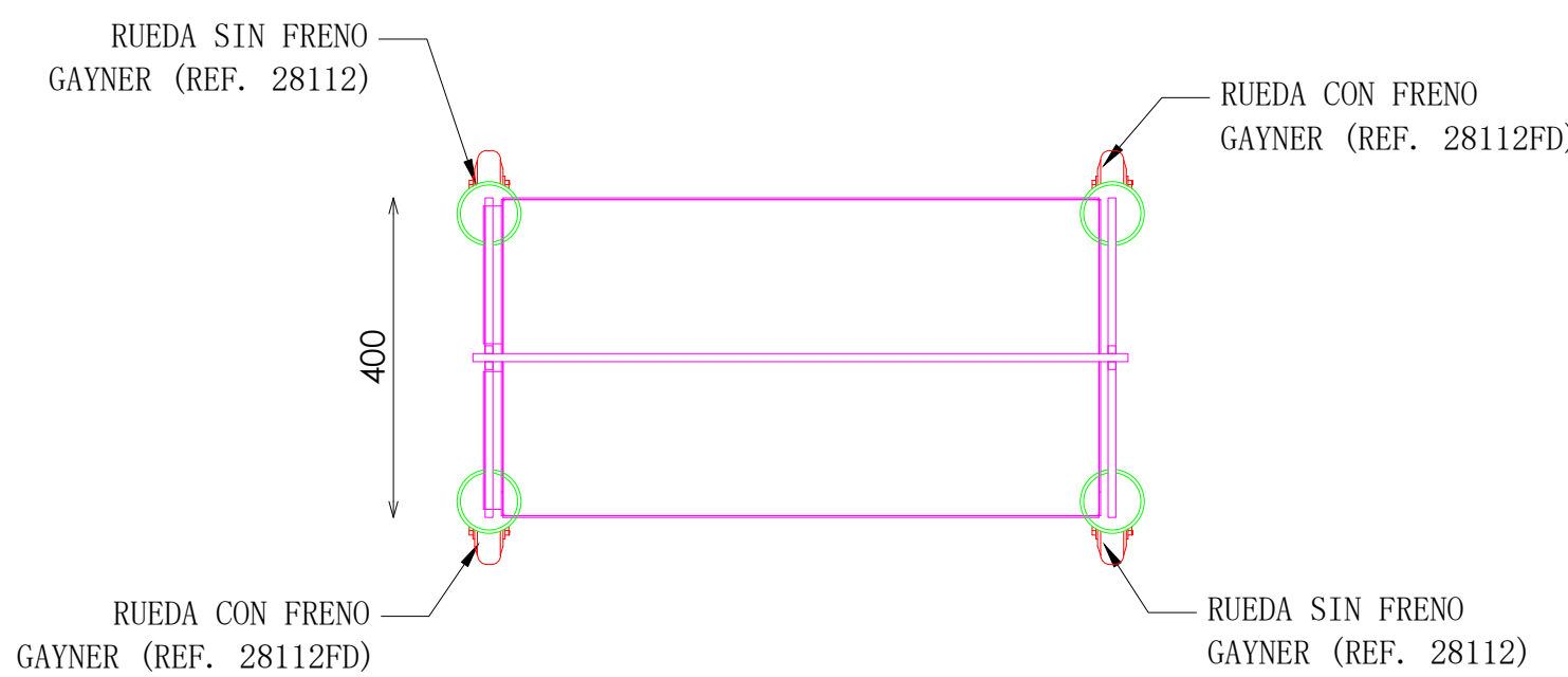
PLANTA
