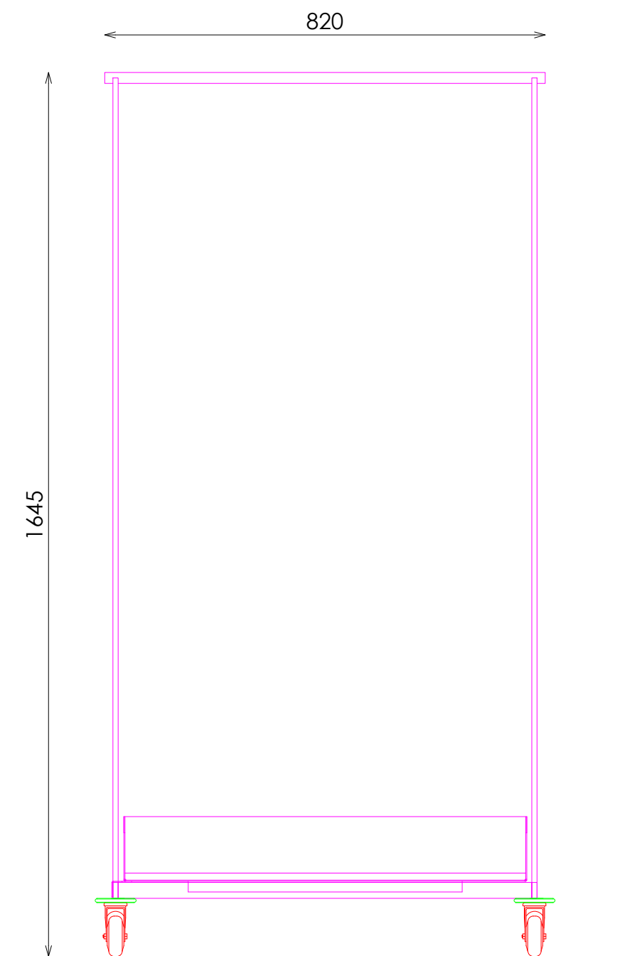
ALZADO
