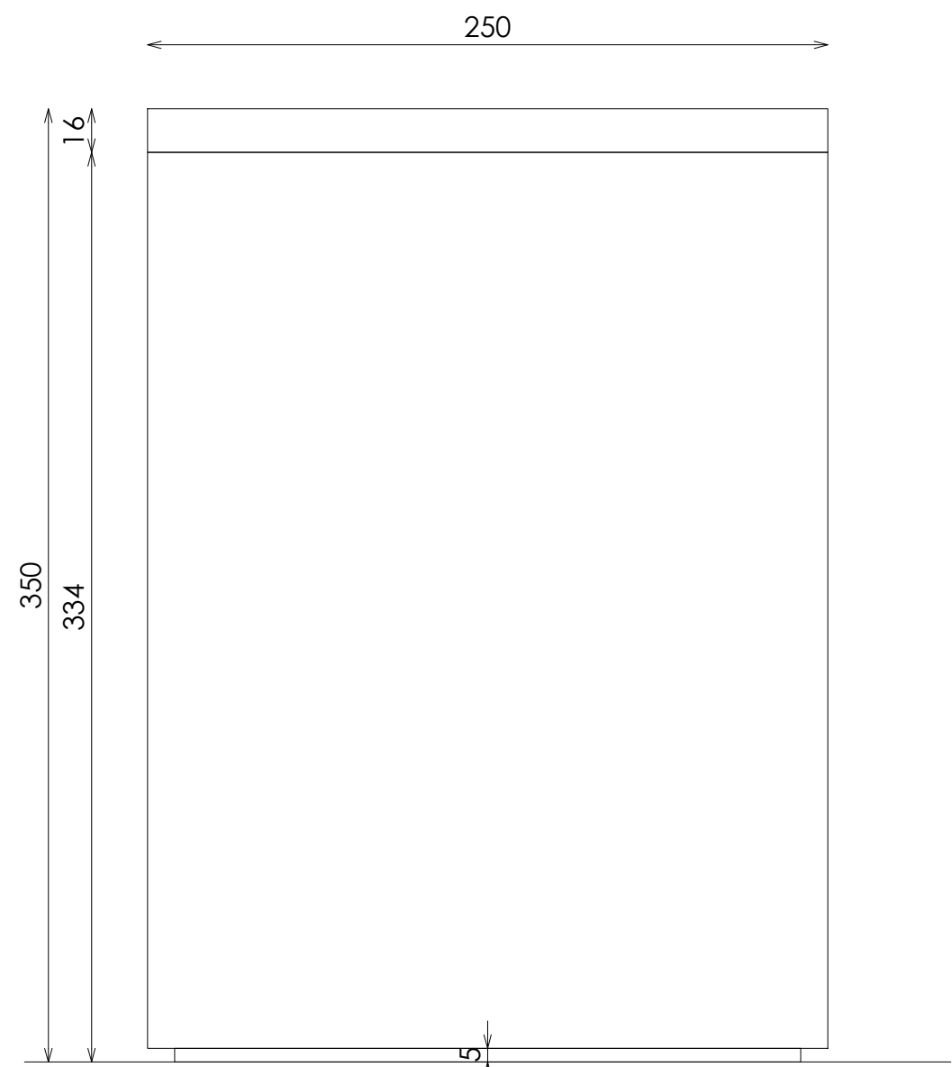
ALZADO
