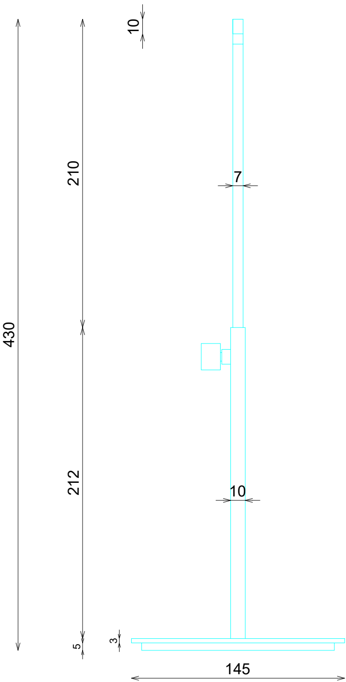
ALZADO
