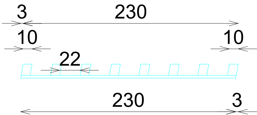
ALZADO
