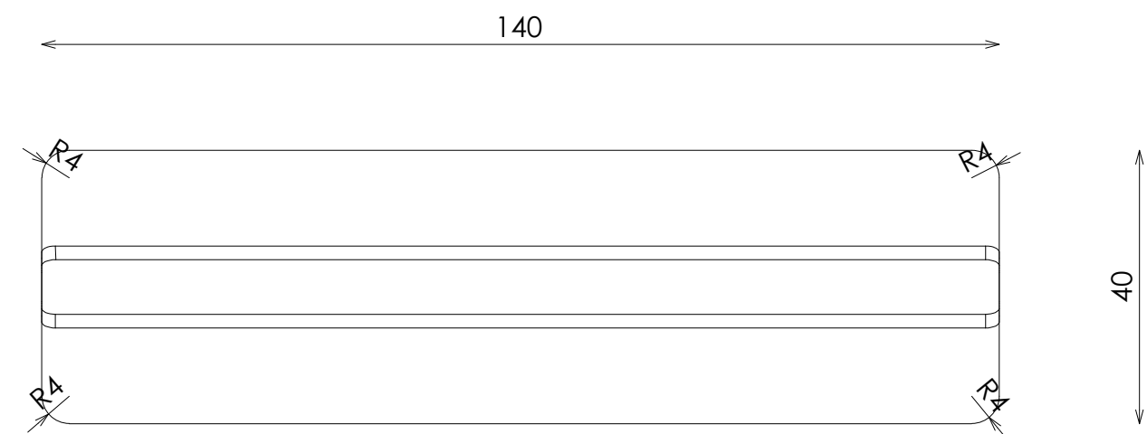
PLANTA
