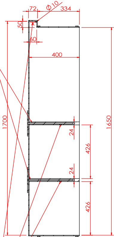
剖面 AG-AG
