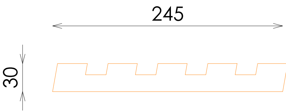
ALZADO
