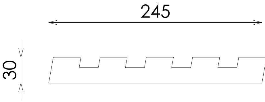
ALZADO
