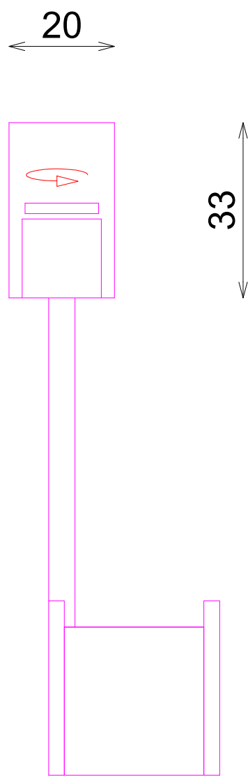
ALZADO
