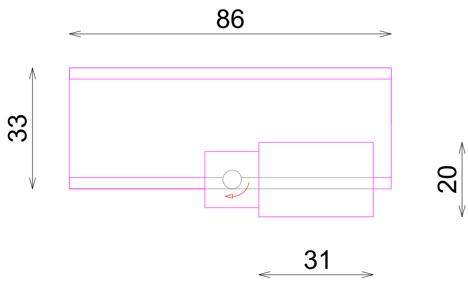
PLANTA POSICION 1
