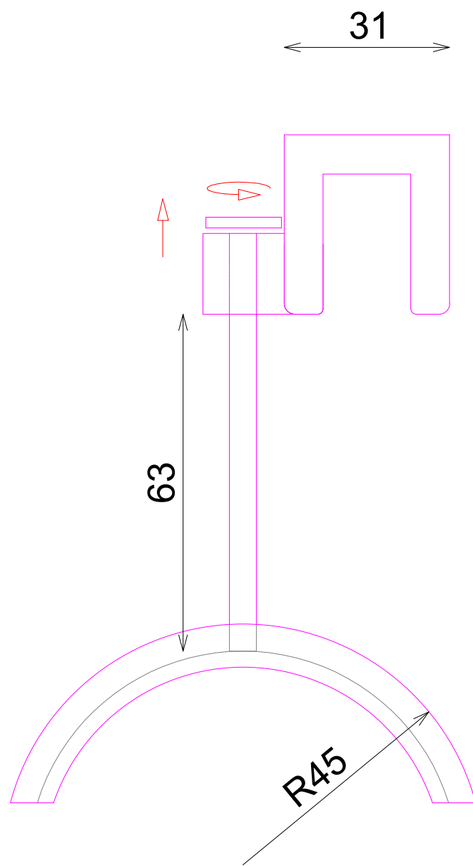
ALZADO
