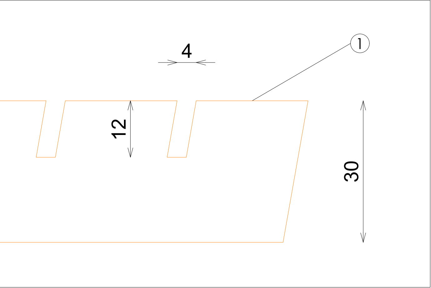
DETALLE BANDEJA
