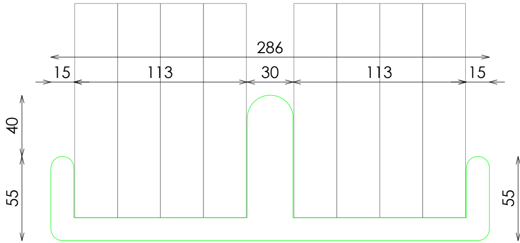
ALZADO
