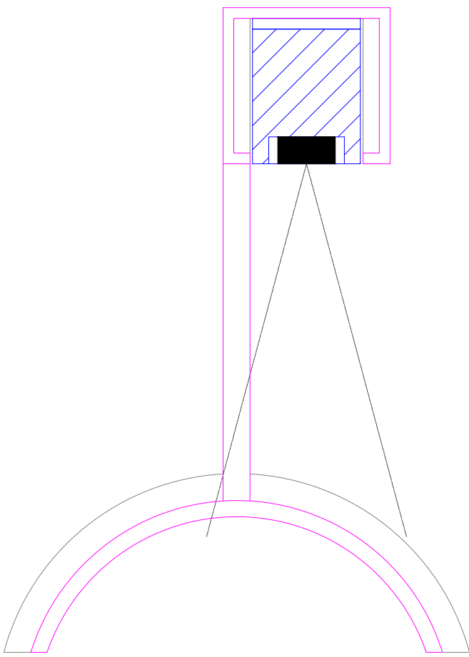
SECCION MONTAJE BARRA 20x25
