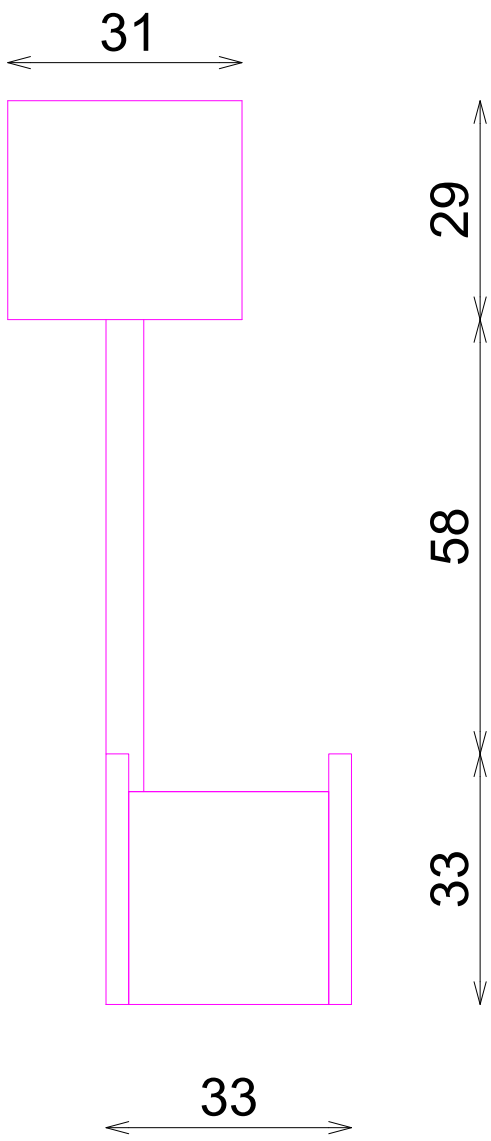
ALZADO
