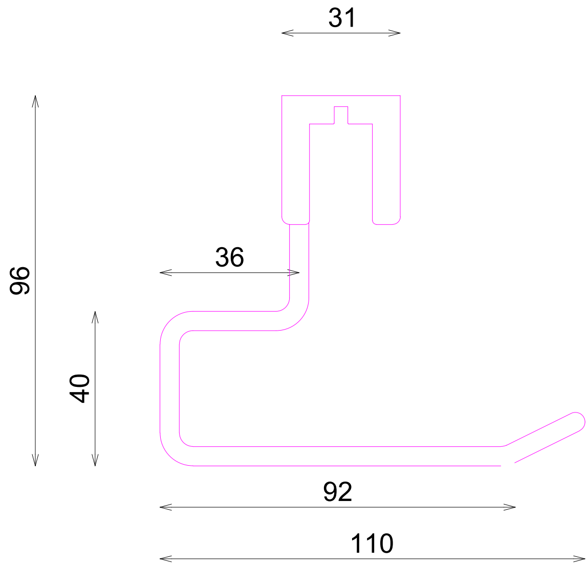
ALZADO
