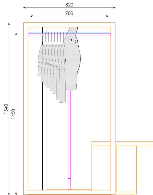
ALZADO IZQUIERDO
