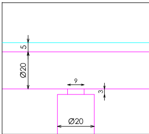
DETALLE C
