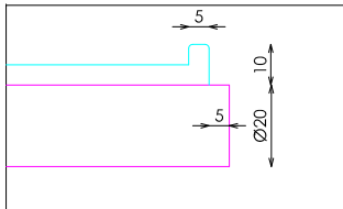
DETALLE ANTIROCE
