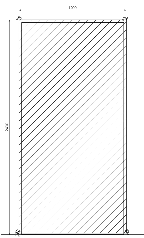
ALZADO
