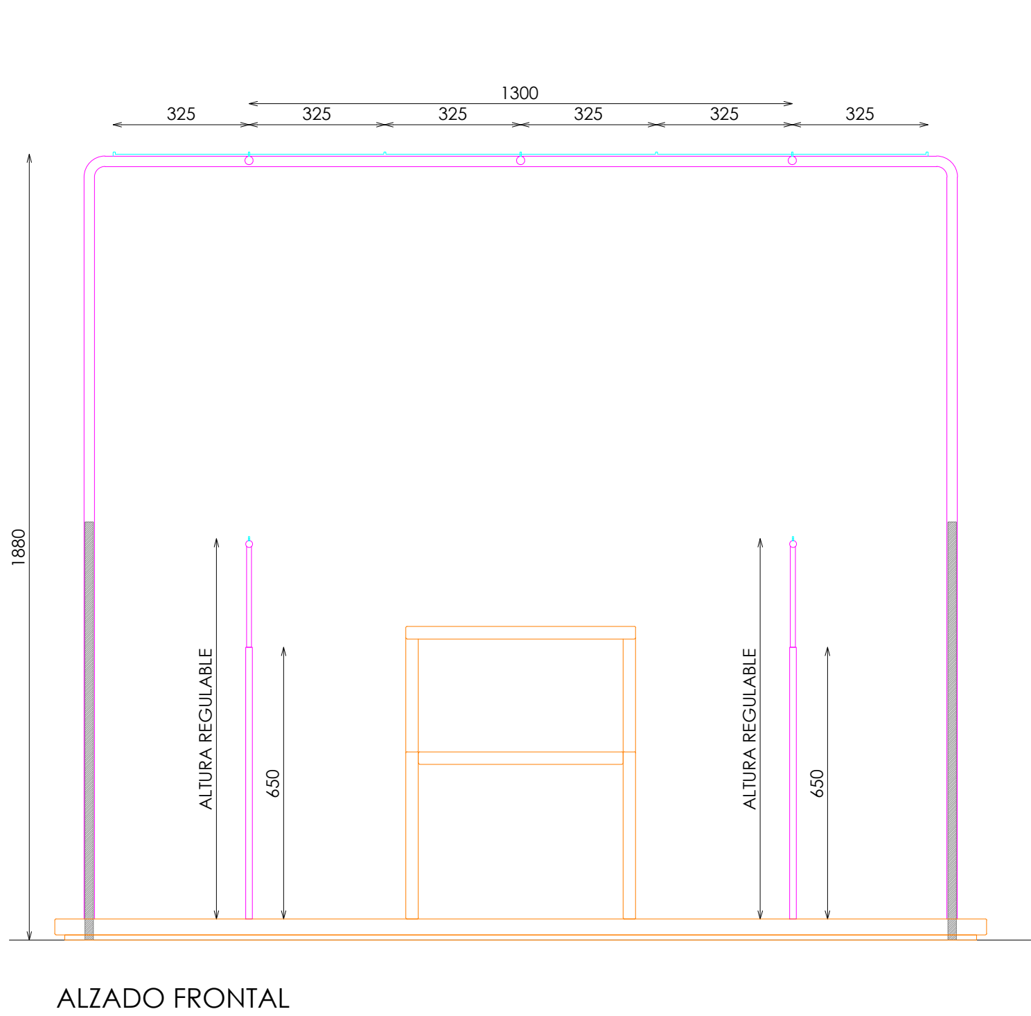
ALZADO FRONTAL
