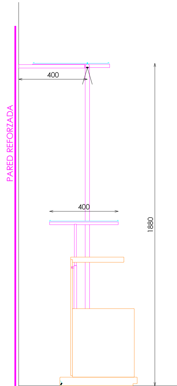
SECCIÓN
