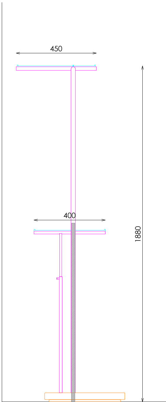
ALZADO LATERAL
