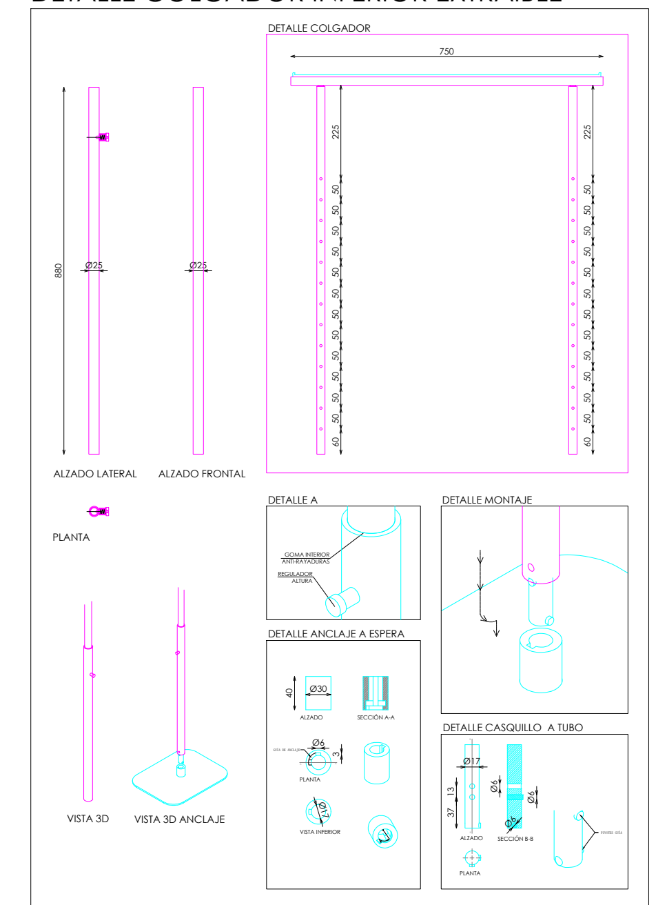
DETALLE COLGADOR INFERIOR EXTRAIBLE
