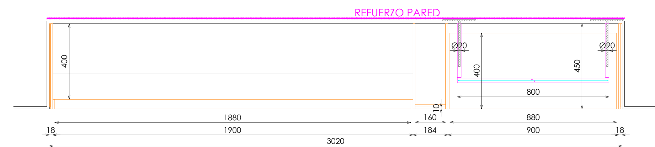
PLANTA
