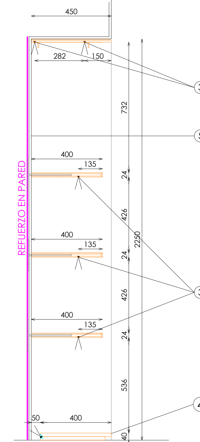
SECCIÓN
